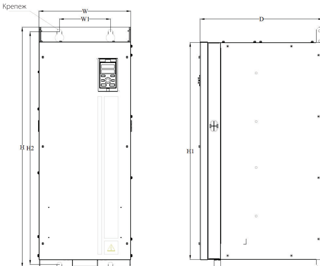
Рис.2-6.8. Чертеж преобразователя частоты типоразмер В8
