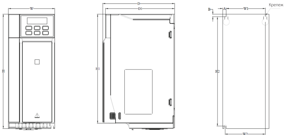
Рис.2-6.2. Чертеж преобразователя частоты типоразмер В2
