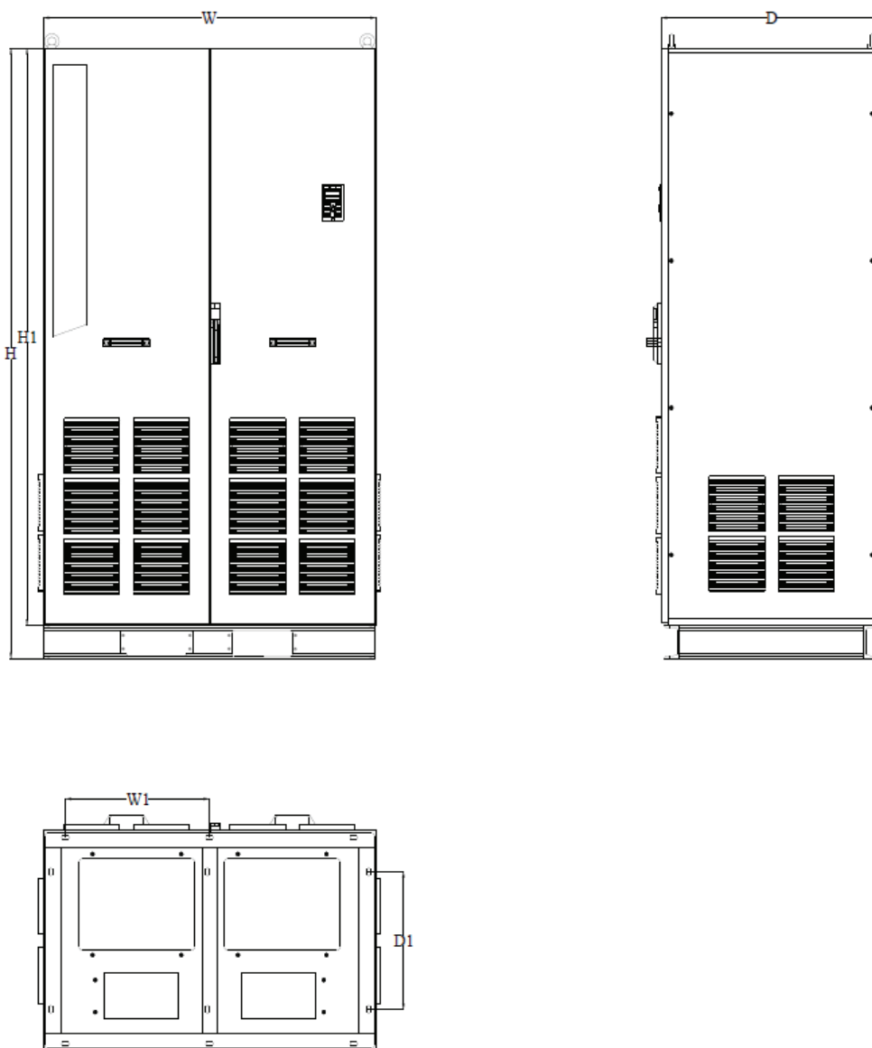
Рис.2-6.12. Чертеж преобразователя частоты типоразмер В12
