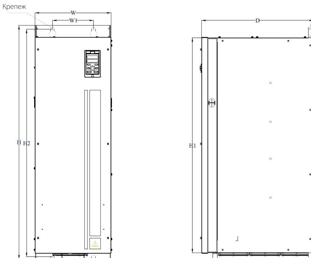
Рис.2-6.9. Чертеж преобразователя частоты типоразмер В9
