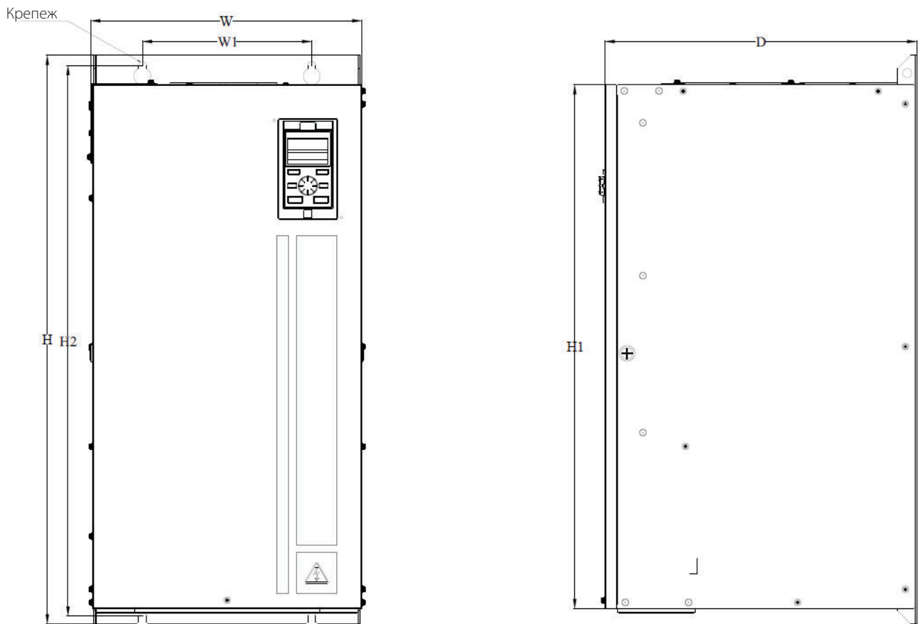
Рис.2-6.7. Чертеж преобразователя частоты типоразмер В7
