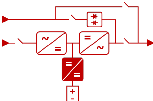
Структурная схема ИБП VEDAUPS
